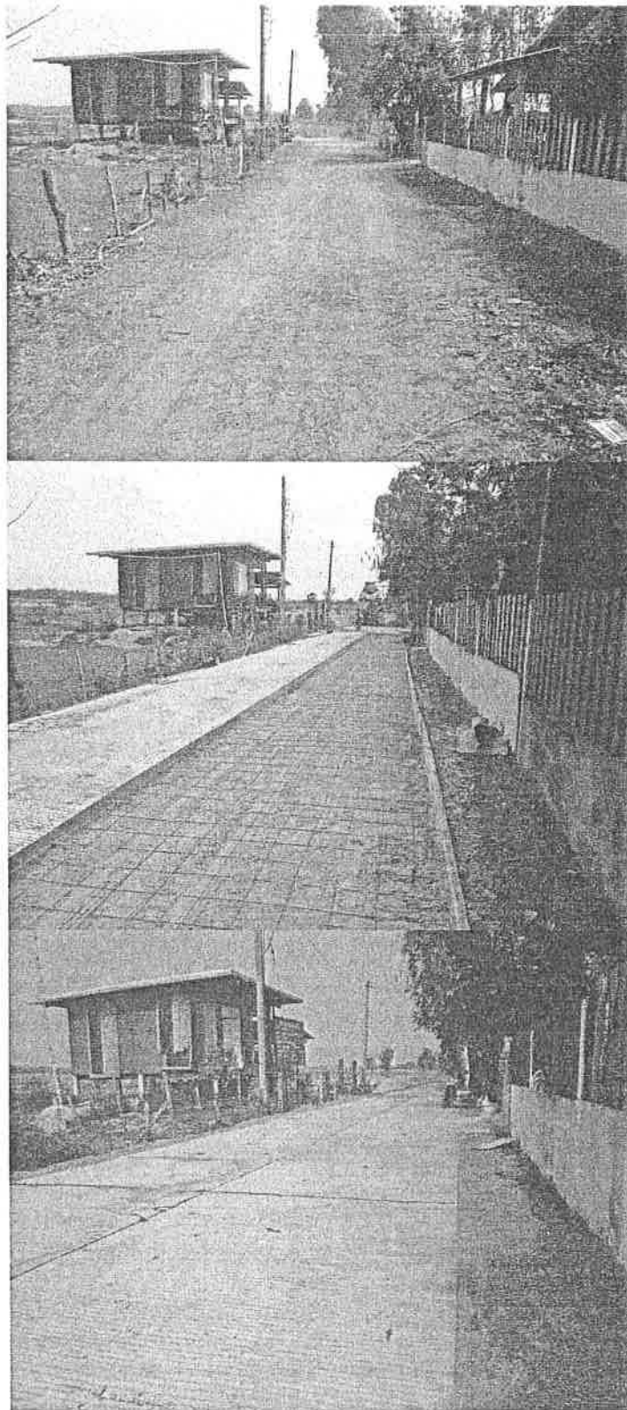
โครงการก่อสร้างถนน คสล. บ้านโพหนอง หมู่ที่ 9 (จากสามแยกบ้านนายทองดำ - สี่แยกบ้านนายบุญทัน)
